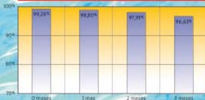
Estabilidad de DOXI-10 PREMIX tras granulación a 80... C y 2,5 atm.
